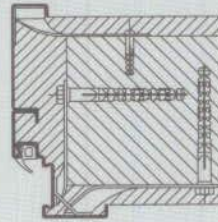
Téglafal fal-típlis-horgony
