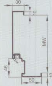
Befoglakók, csavarozható
