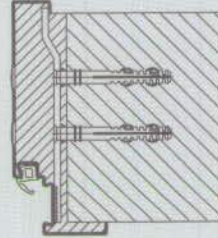
Nyers téglafal vagy beton tıplis szerelés a tok kávjáján keresztül 205 mm pótaszélességig
