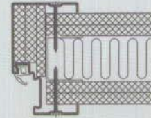
Csavarozott szerelés
