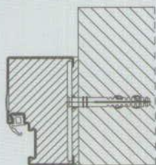
Tıplis szerelés a tok nyílása felıl
