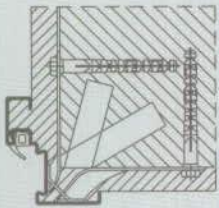
Téglafal fal-típlis-horgony
