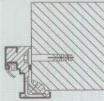
Nyers téglafalba vagy betonba szerelőlemez a rejtett szereléshez
