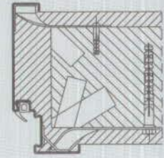
Téglafal fal-típlis-horgony
